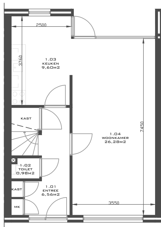
BEGANE GROND
